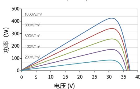
功率-电压曲线 (425W)
